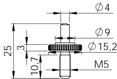
Höhenverstellungsschraube level adjustable screw
