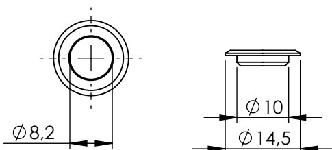
Bundscheibe Step washer
